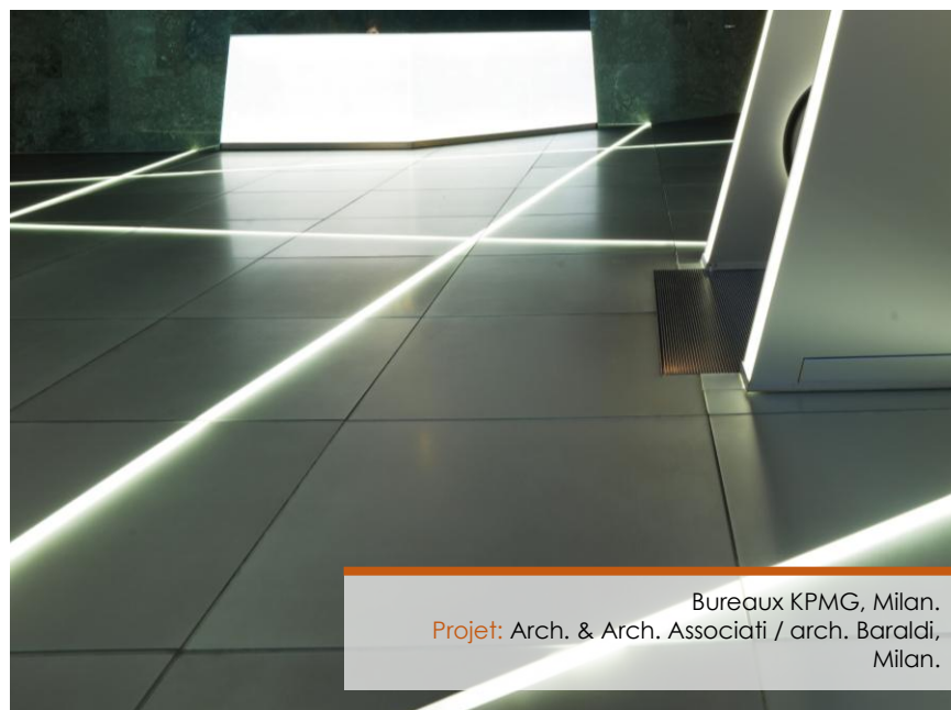
Marches en verre antidérapant : composition de haut en bas: Madras® Pixel Flooring 8 mm extraclair, feuilleté PVB transparent, float extraclair 8 mm, PVB transparent, float extraclair 8 mm.
